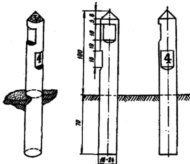
Рис. 5. Столб граничный
