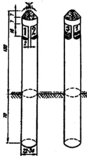
Рис. 3. Столбы квартальные деревянные
