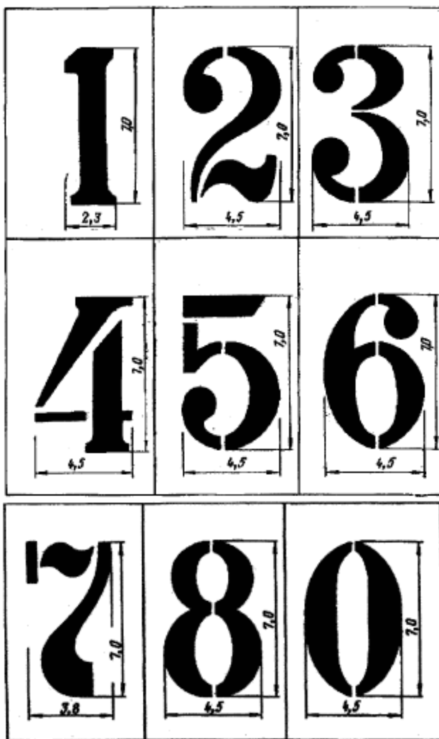
Рис. 1. Трафареты для квартальных столбов
