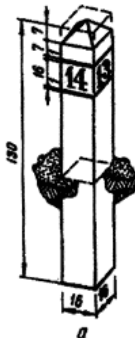
Рис. 2. Столб квартальный железобетонный
